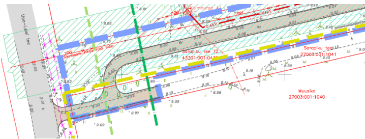
Joonis 1. Kooskõlastatud ristumiskoha lahendus (km 0,232)
